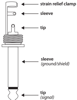
Abb. 4.2: 6,3 mm-Monoklinkenstecker
