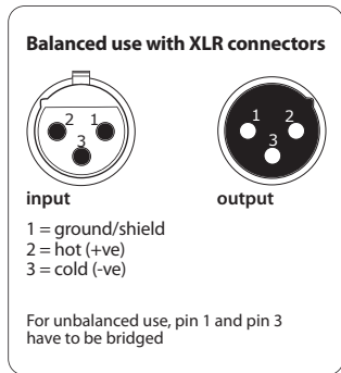
Fig. 4.1: Ligações XLR
